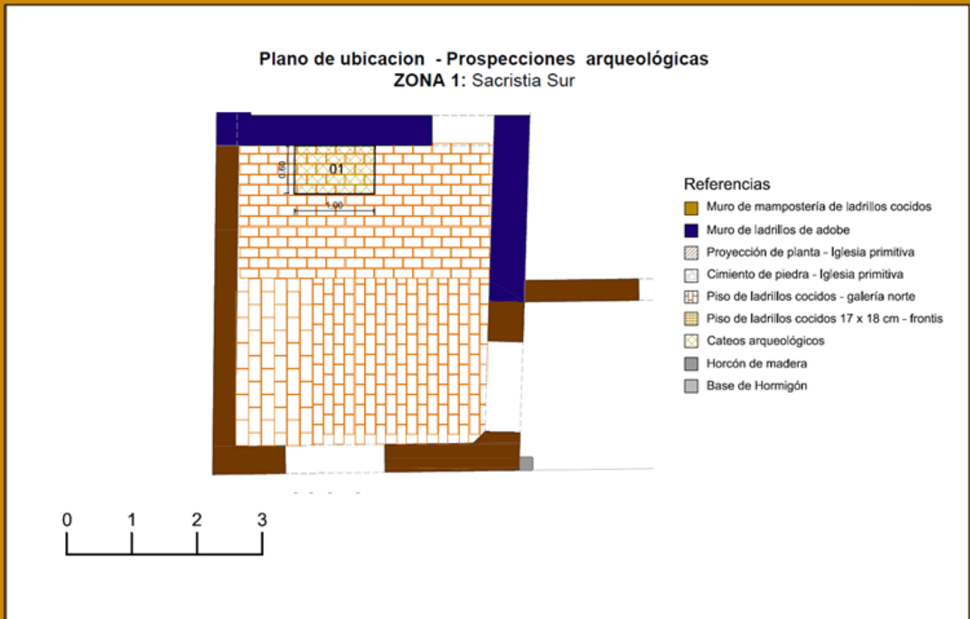
Fig. 4.6. Ubicación calicata Sacristía Sur, y tipos de pisos. También se observan parte de los muros de ladrillo de adobe y el de mampostería de ladrillo cocido
