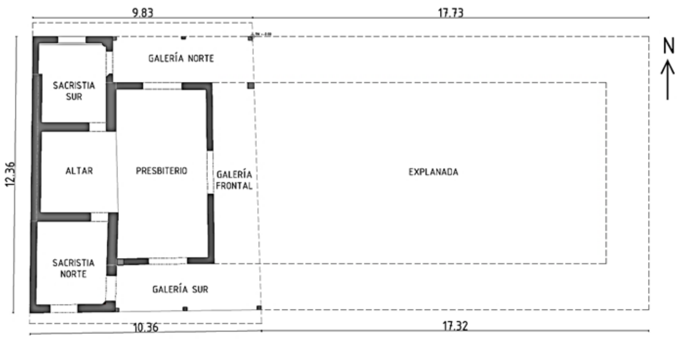
Fig.2.8. Planta del conjunto de la Iglesia, donde se observa el área de la Iglesia antigua, configurado estructuralmente a partir de materiales reciclados de la Iglesia Primitiva. El sector denominado “explanada” es la antigua nave central de la Iglesia de 1844, la cual fue demolida.
