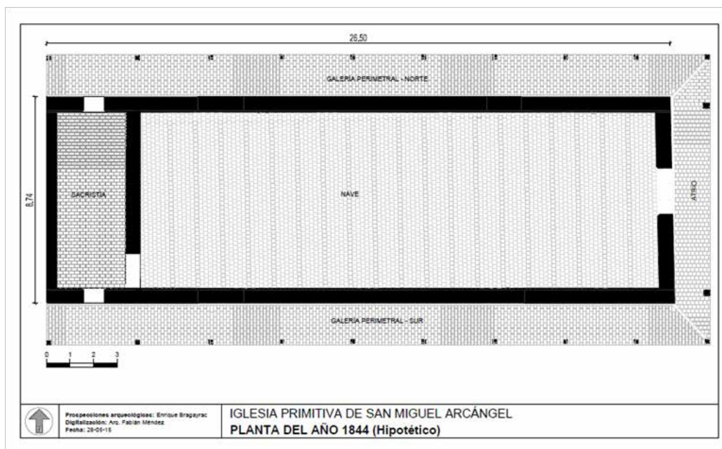
Fig. 6.2 Planta de la Iglesia Primitiva del año 1844.
