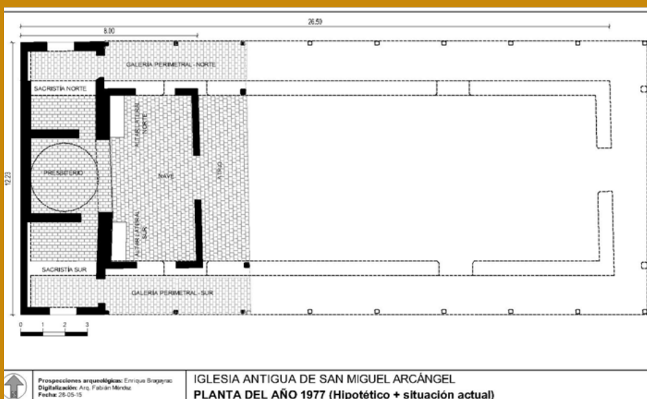
Figura 6.4. Planta de la Iglesia Primitiva completamente modificada para el año 1977, donde se configura un oratorio por las dimensiones que presenta, después de la demolición.
