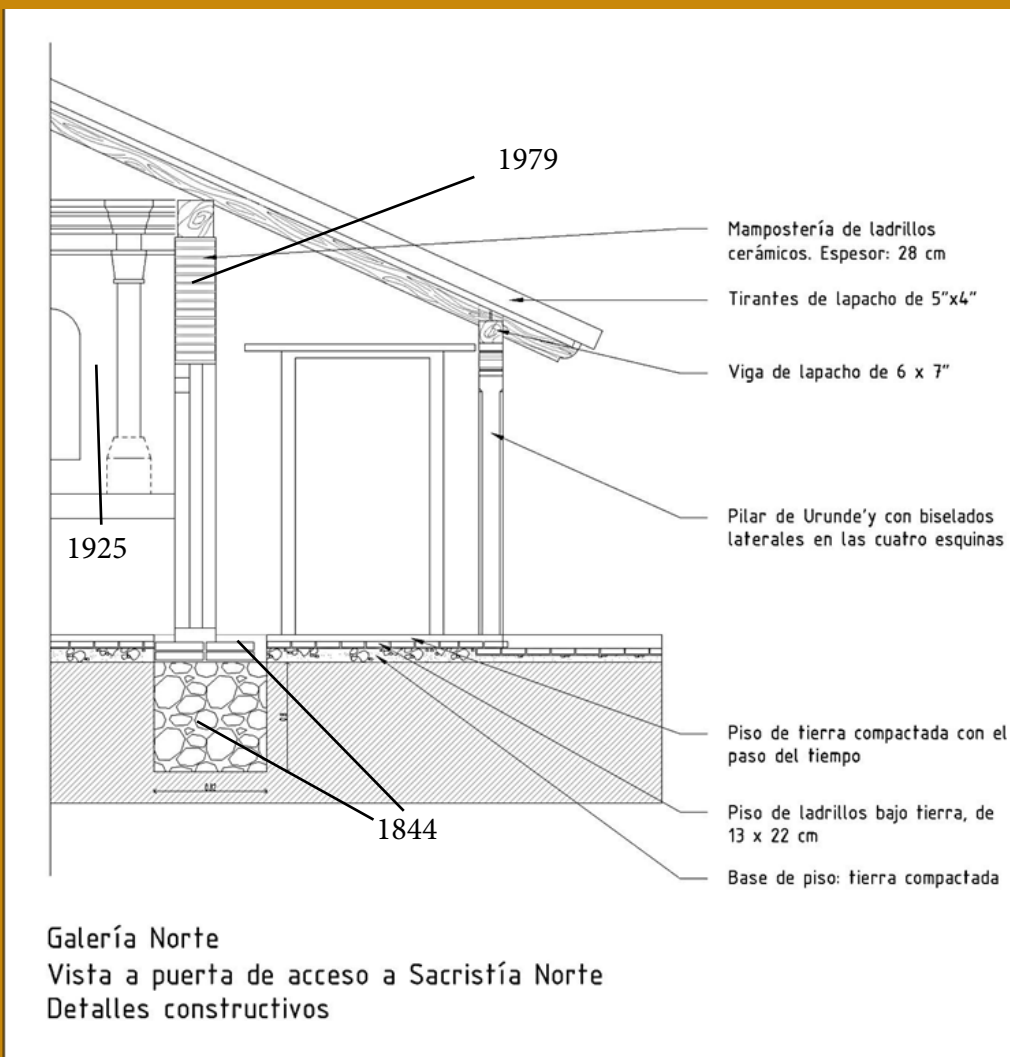
Fig. 6.5. Corte de la galería Norte, indicando los horizontes constructivos y materiales utilizados, así como los años de edificación.
