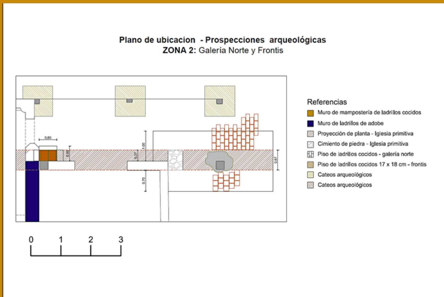
Fig. 4.17. Plano de localización de los cateos realizados, en función a las intervenciones a realizar para su puesta en valor. Aquí podemos observar en color rojo evidencias de la nivelación de adobes sobre un cimiento de piedra correspondiente a la iglesia primitiva. Así mismo, se puede observar los testimonios de los tipos de pisos originales, tanto para la galería sur como la galería del frontis de la iglesia antigua.
