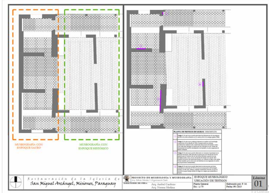
Fig. 6.1 Planta hipotesis de proporción aurea – Iglesia Primitiva 1844/1853
