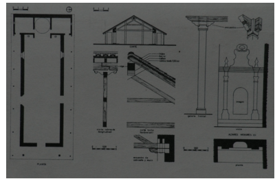
Planos del viejo templo de San Miguel.
